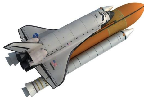
космический шаттл
