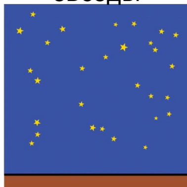
ЗВЕЗДЫ
