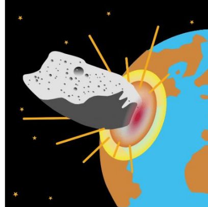
МЕТЕОРИТ
