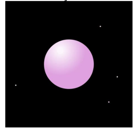
Плутон
