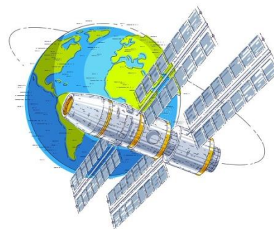
космический аппарат
