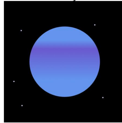
Нептун
