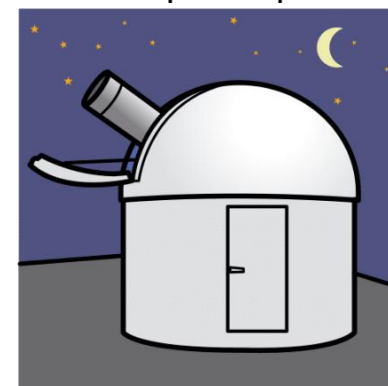
ОБСЕРВАТОРИЯ
