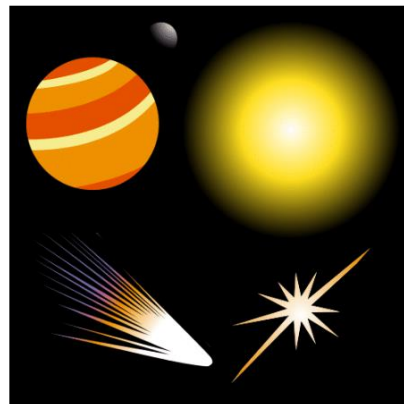
ТЕЛЕСКОП
