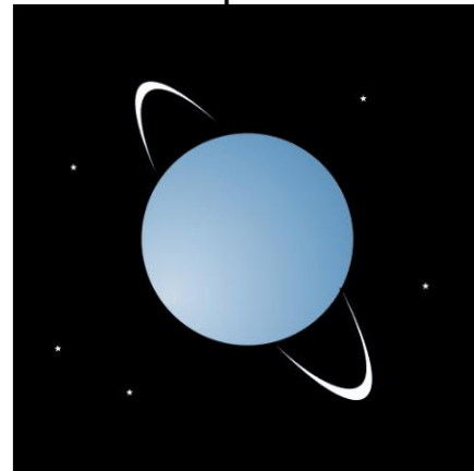
Уран
